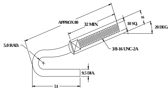
STUD DETAIL
